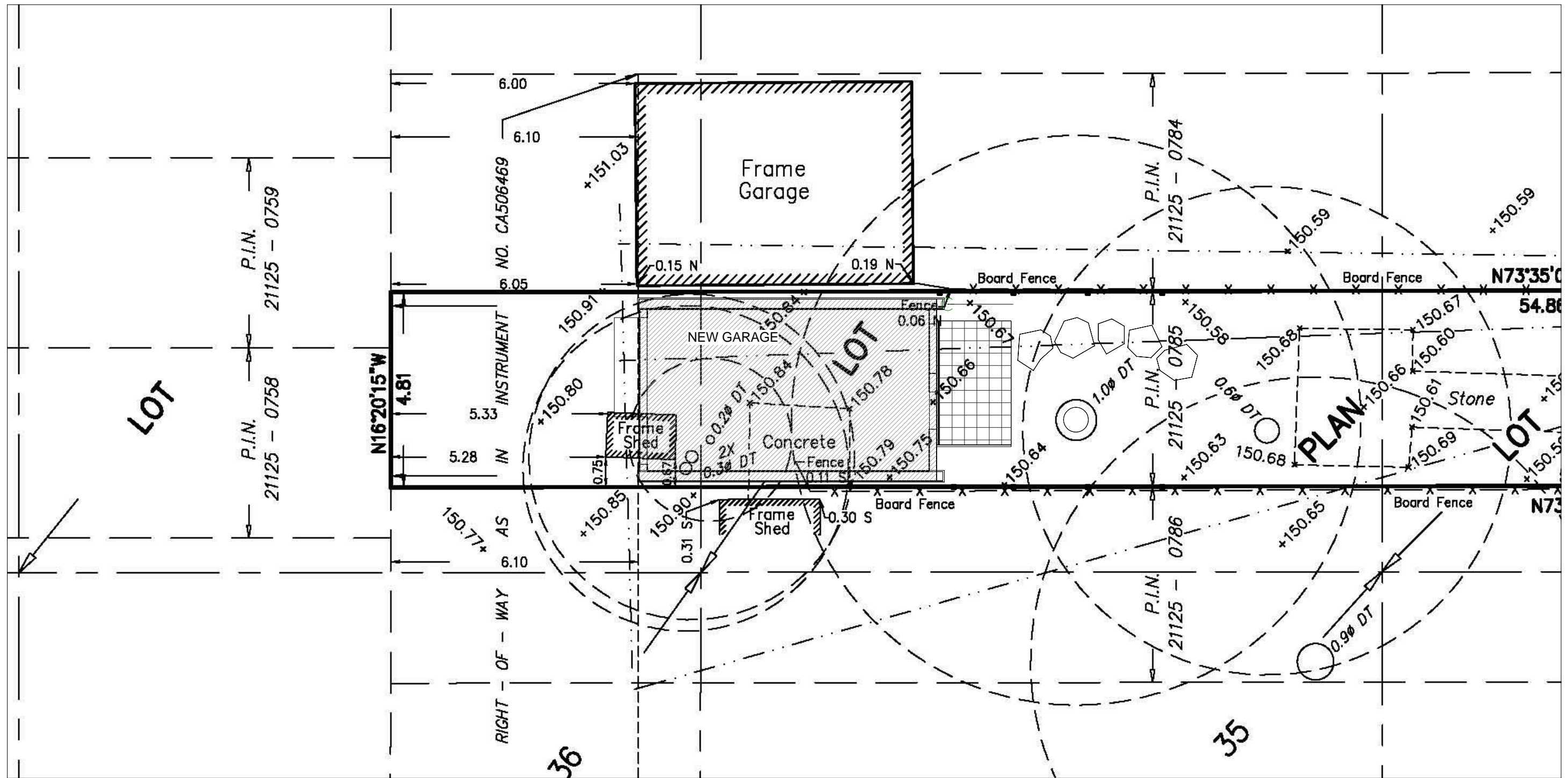
① Partial Site Plan 1:100
