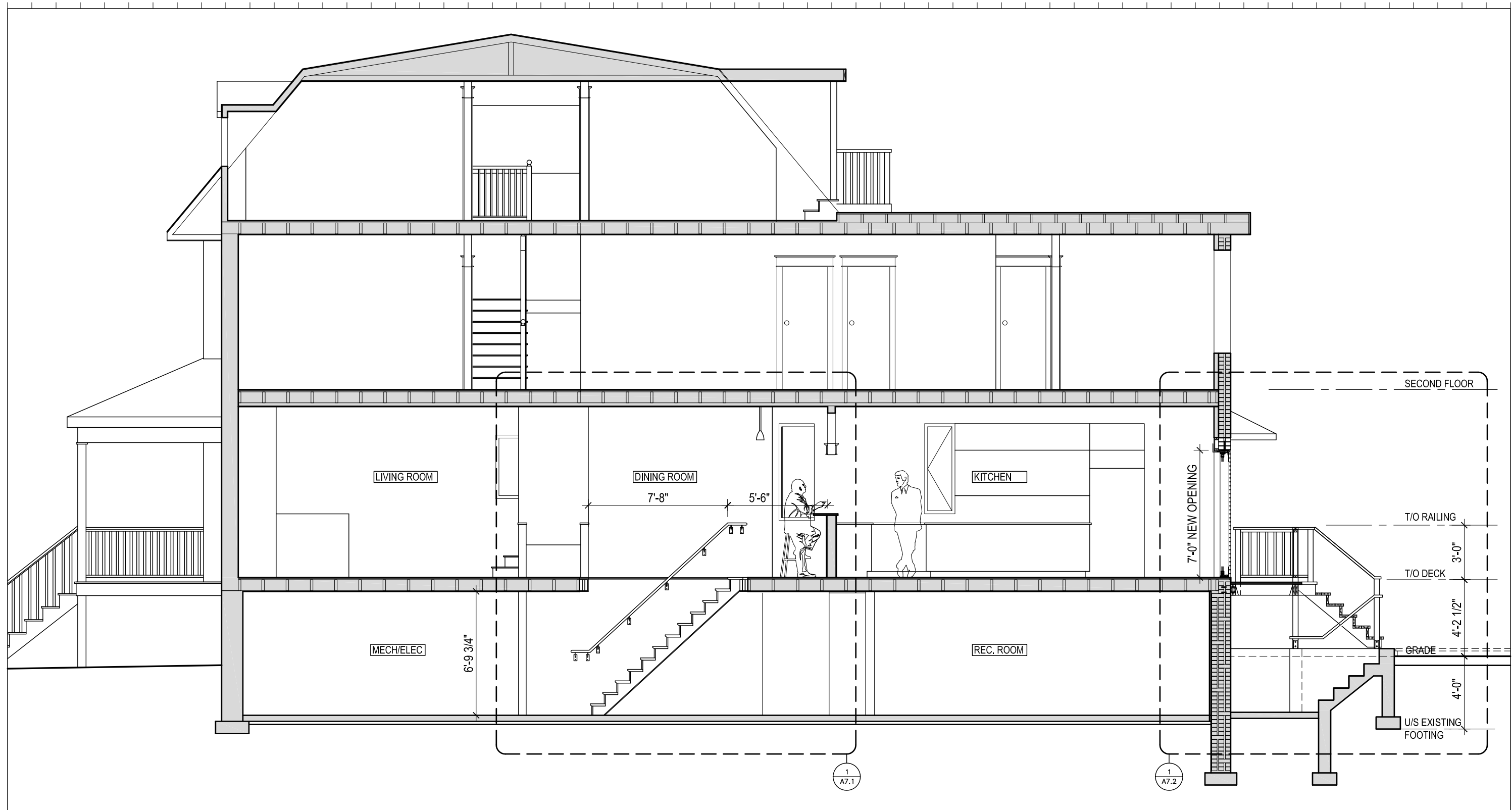
1 Section A A8 Scale: 3/16"=1'-0"
