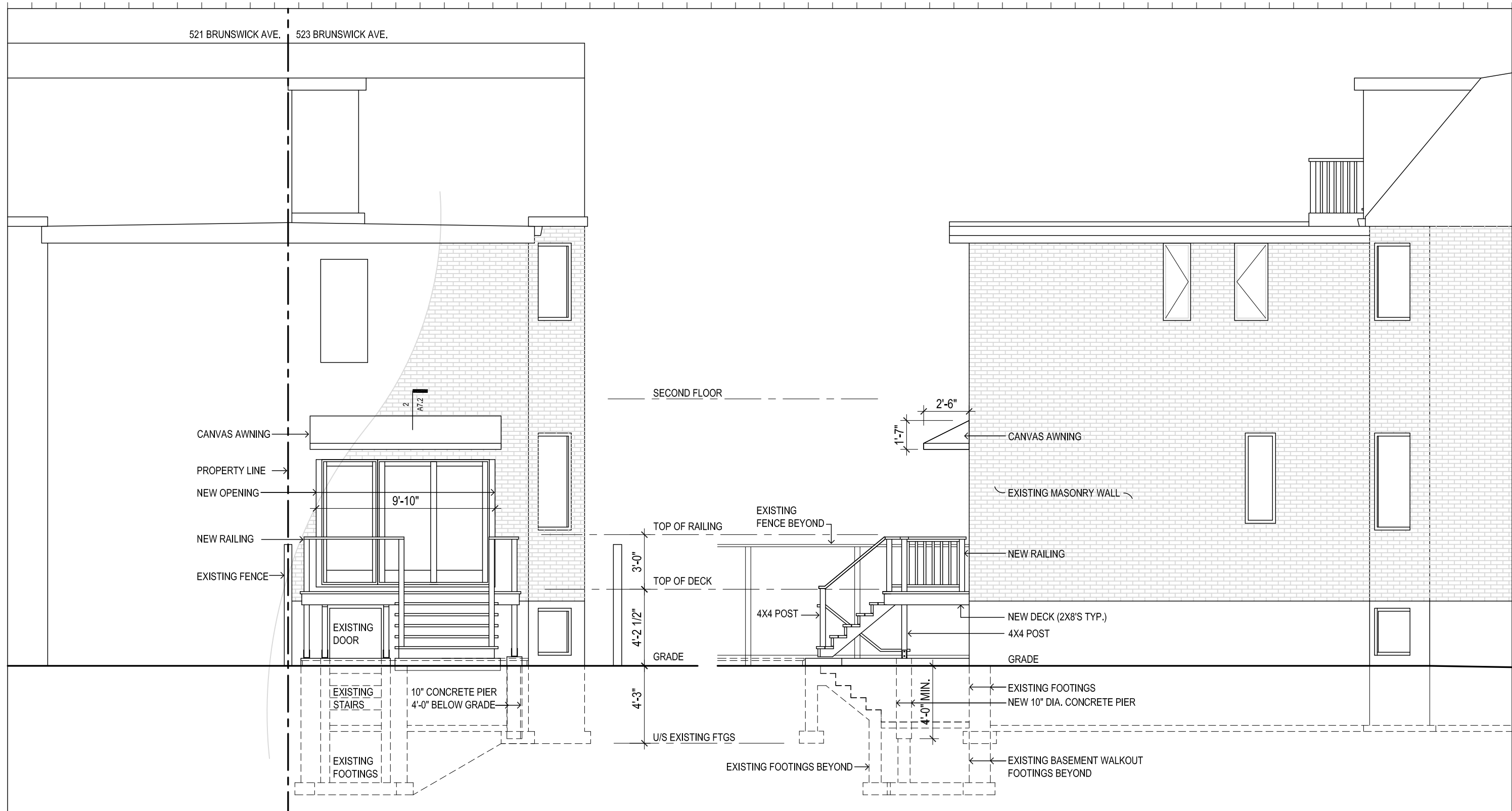
2 West Elevation A6 Scale: 3/16"=1'-0"
