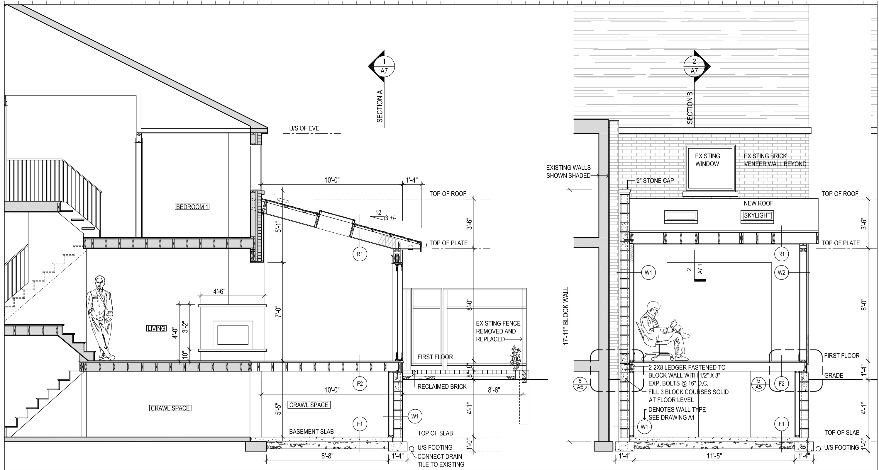
SECTION B Scale: 1/4"=1'-0"
