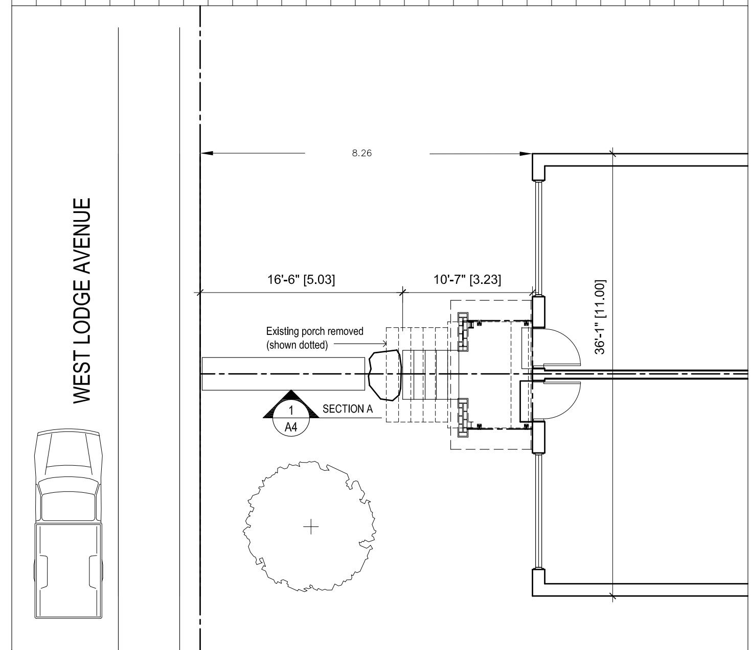
1 SITE PLAN A1 Scale: 1/8" = 1'-0"
