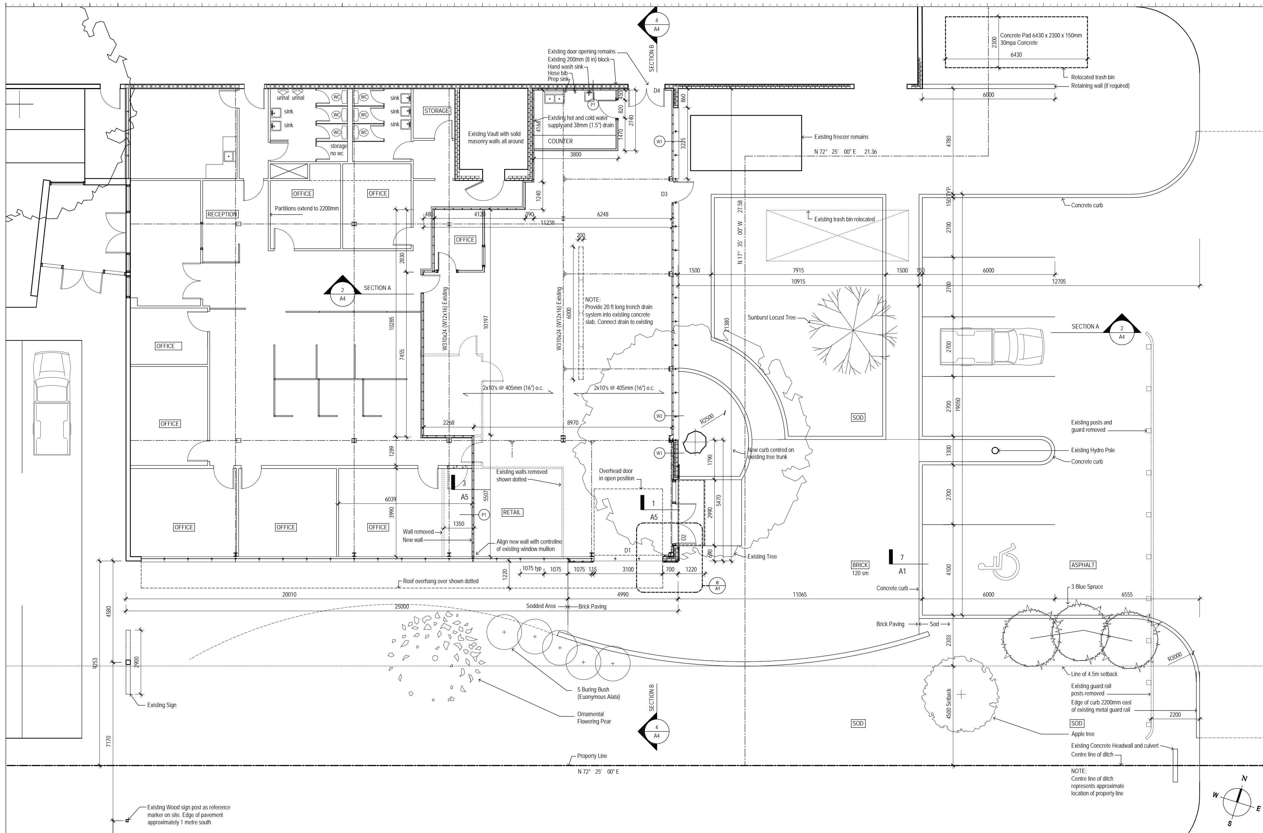
1 FLOOR PLAN A2 Scale: 1:100
